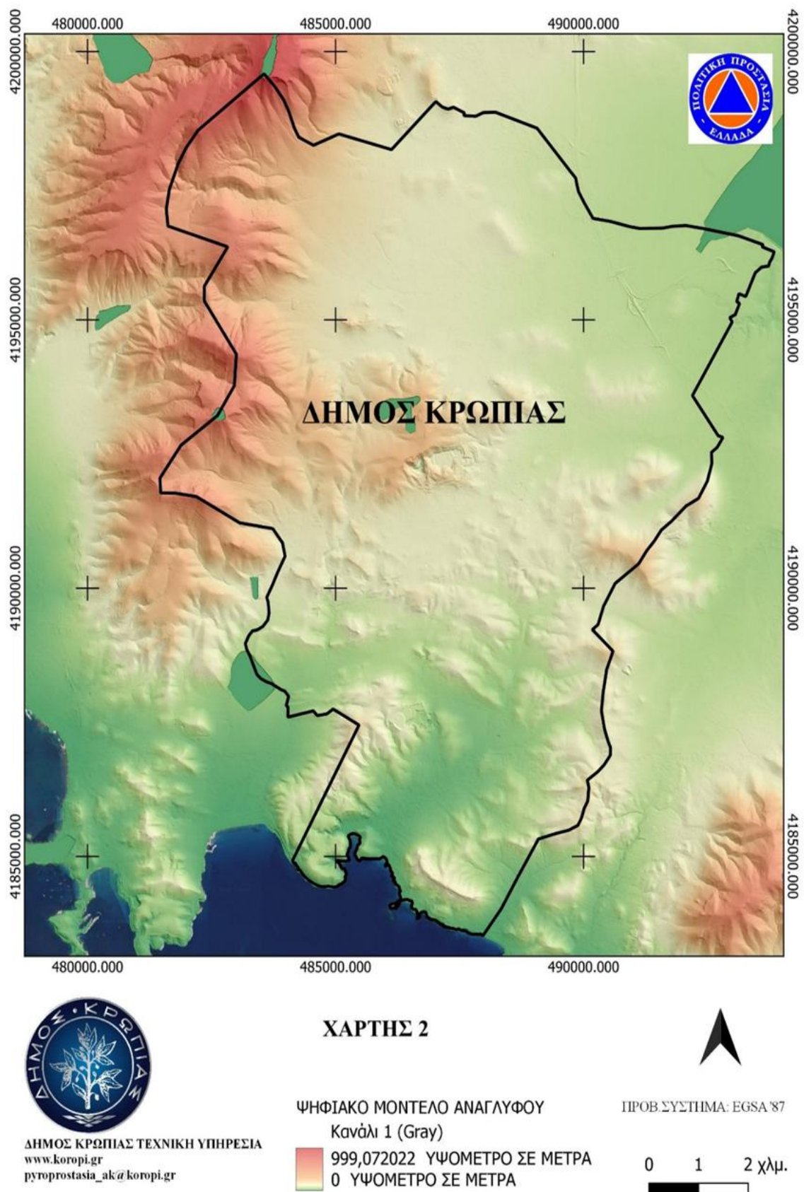
Εικόνα 5: Ψηφιακό Μοντέλο Αναγλύφου DEM Δήμου Κρωπίας.
