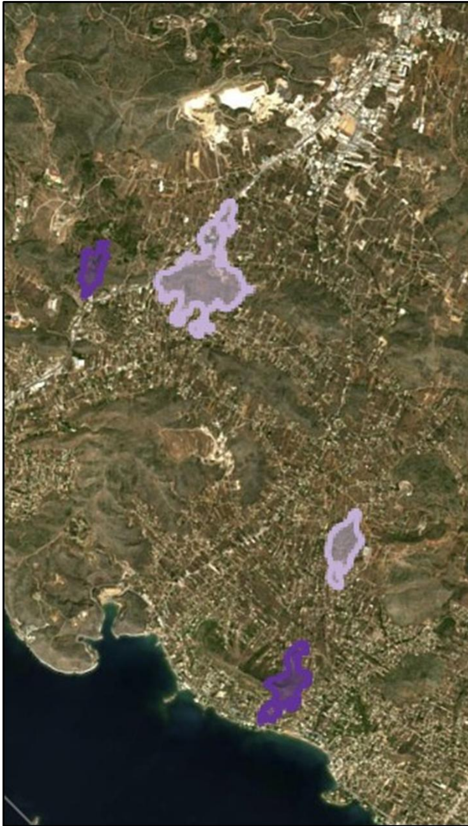
Εικόνα 9: Καμμένες εκτάσεις ( ροζ επιφάνεια 2024, μοβ επιφάνεια 2025), πηγή https://www.copernicus.eu/en
