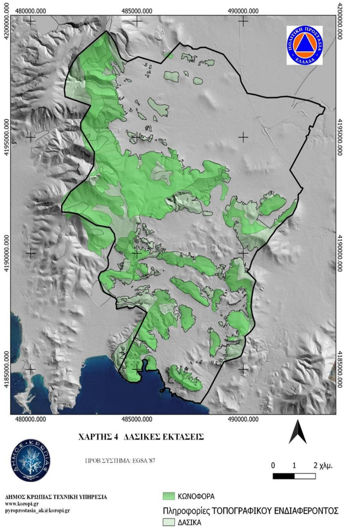
Εικόνα 6: Δασικές Εκτάσεις – Εκτάσεις Κωνοφόρων.
