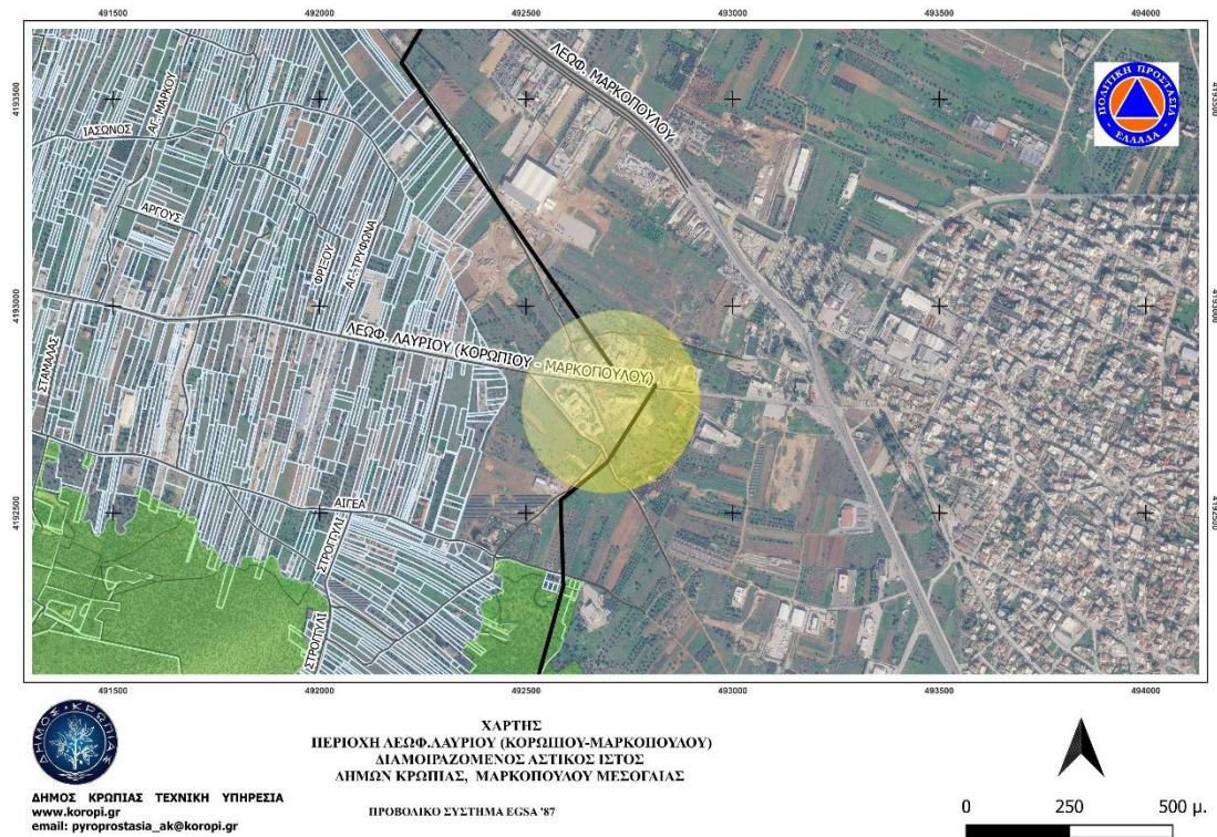
Εικόνα 27: Διαμοιραζόμενος Αστικός Ιστός (κίτρινες επιφάνειες) με το Δήμο Μαρκοπούλου
